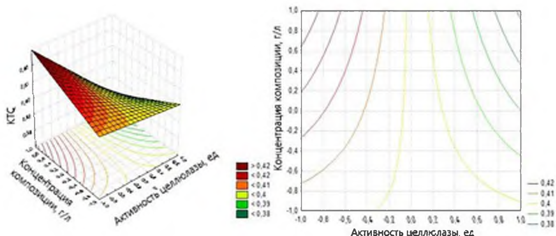
Рисунок 4 – Графическая зависимость коэффициента тангенциального сопротивления трению хлопчатобумажной ткани от концентрации композиции и активности ферментной составляющей в пропиточной ванне
