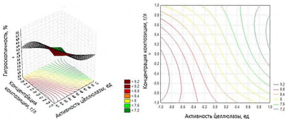
Рисунок 2 – Графическая зависимость гигроскопичности хлопчатобумажной ткани от концентрации композиции и активности ферментной составляющей в пропиточной ванне
