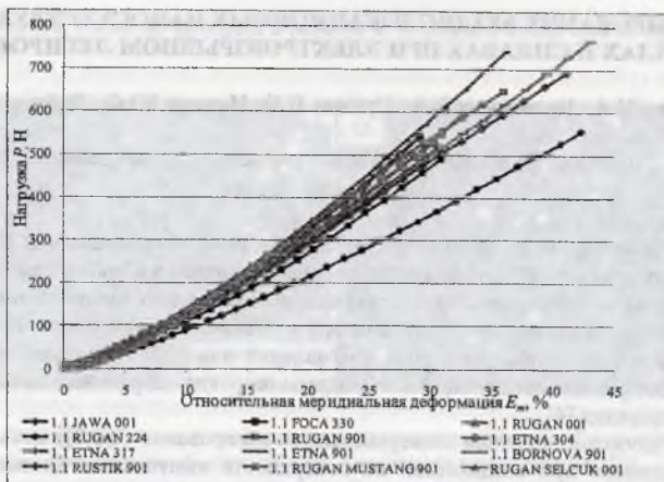
Рис. 1. Кривые зависимости нагрузки от относительной меридиальной деформации при двухосном растяжении
