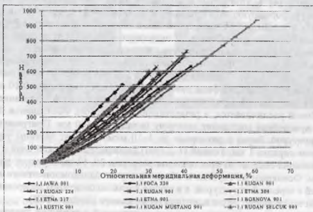
Рис. 2. Кривые зависимости нагрузки от относительной меридиальной деформации при двухосном растяжении после 15% деформирования
