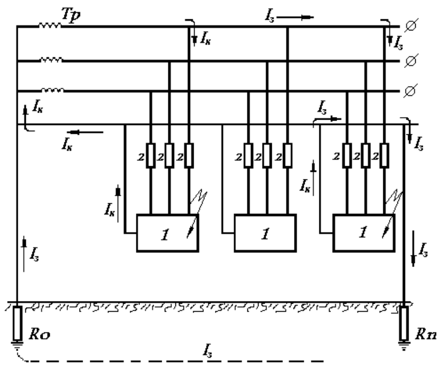
Рисунок 5.1 – Принципиальная схема зануления: 1 – корпус электроустановки; 2 – аппараты защиты от токов короткого замыкания; R_0 – сопротивление заземления нейтрали источника тока; R_n – сопротивление повторного заземления нулевого провода; I_k – ток короткого замыкания при неповрежденном нулевом проводе; I_3 – ток короткого замыкания при обрыве нулевого провода в сети с повторным заземлением нулевого провода
