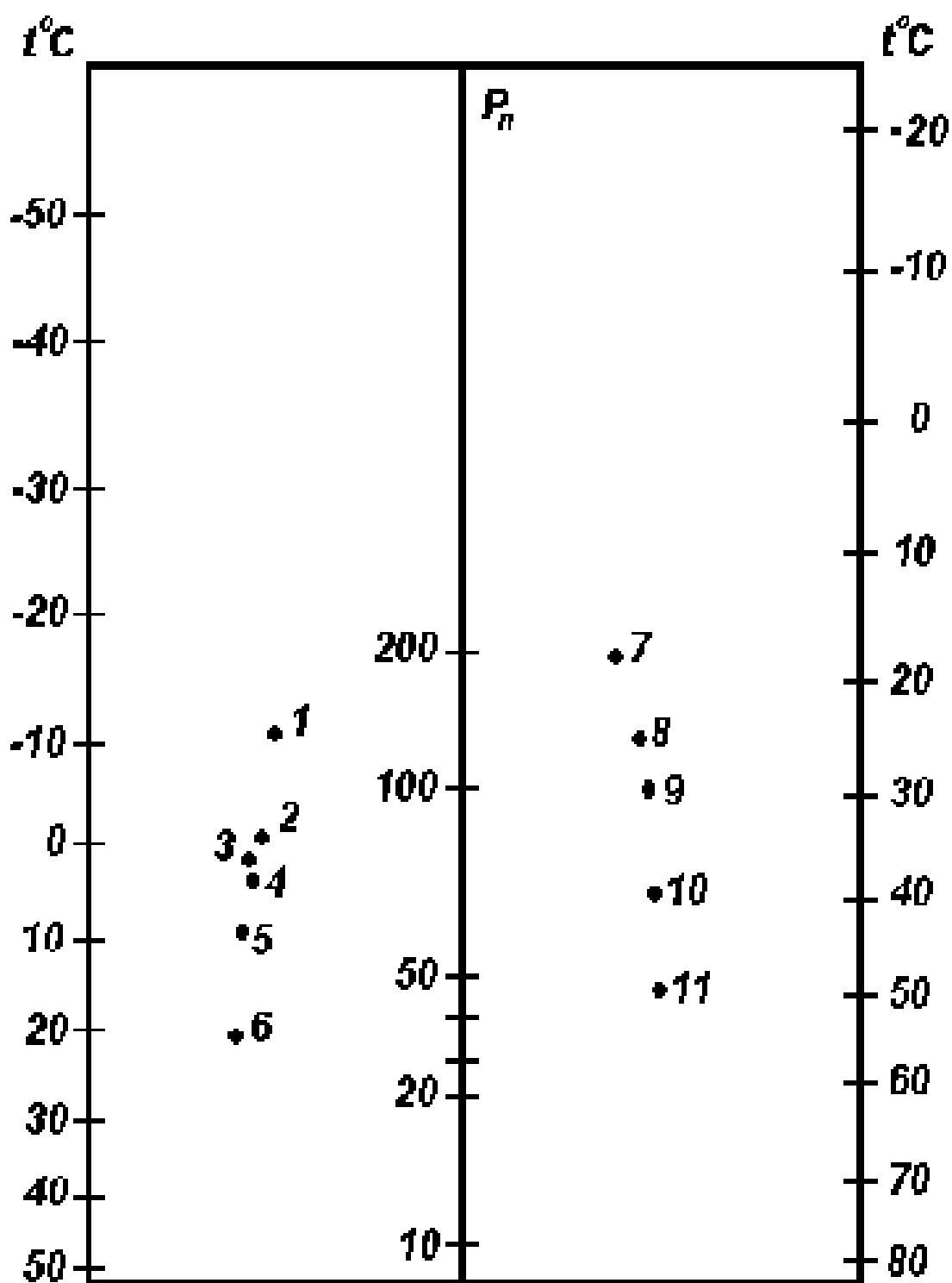
Рисунок 9.1 – Номограмма для определения параметров насыщенного пара горючих жидкостей
