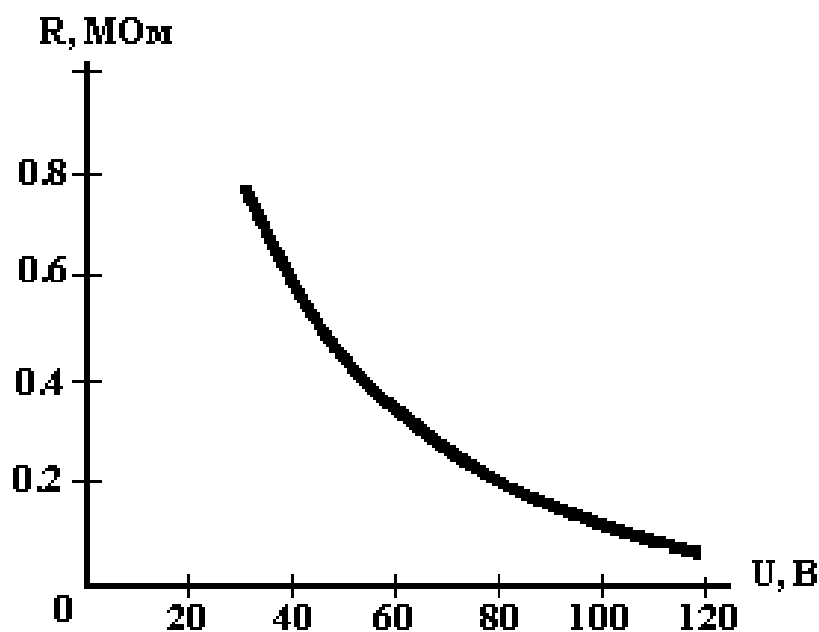
Рисунок 7.1 – Зависимость сопротивления изоляции R_{из} от приложенного напряжения U
