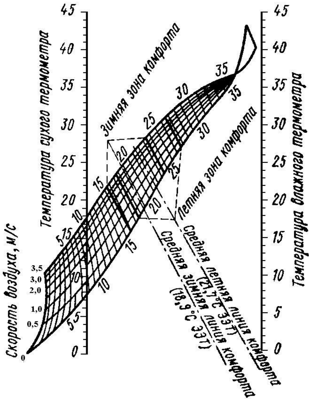
Рисунок 1.1 – Номограмма эквивалентно-эффективных температур
