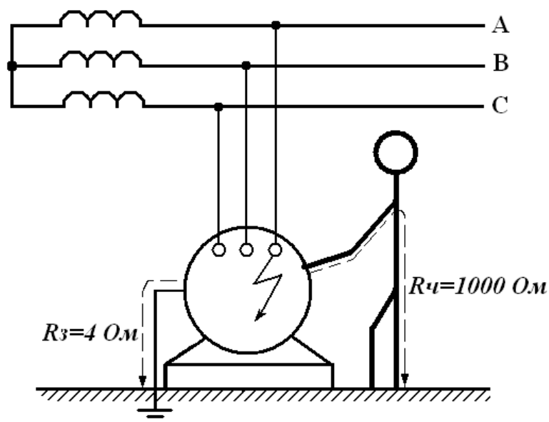
Рисунок 6.1 – Схема защитного заземления: R_z – сопротивление защитного заземления; R_{ч} – сопротивление человека
