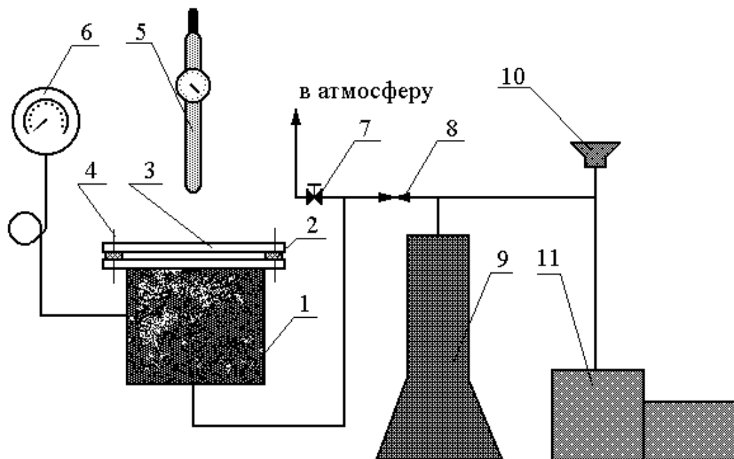
Рисунок 10.1 – Схема экспериментальной установки для исследования герметичности фланцевых соединений: 1 – экспериментальный аппарат; 2 – прокладка из исследуемого материала; 3 – плоский фланец; 4 – болт; 5 – динамометрический ключ; 6 – образцовый манометр; 7 – клапан; 8 – вентиль; 9 – ресивер; 10 – регулятор давления; 11 – компрессор
