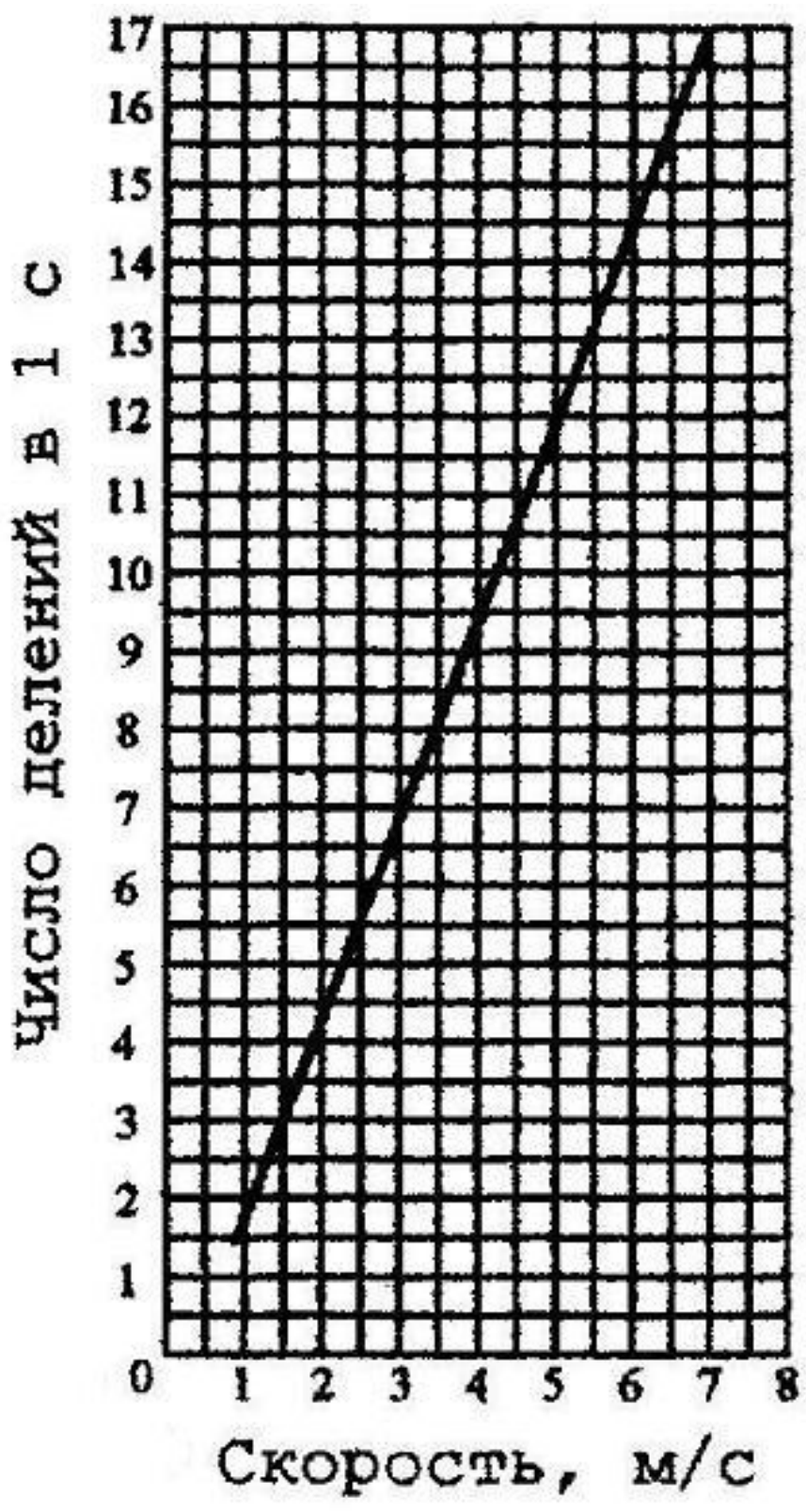
Рисунок 1.3 – Тарировочный график для определения скорости движения воздуха анемометром
