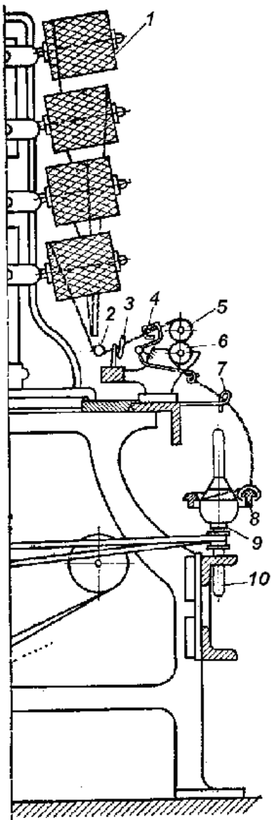
Рисунок 9 - Технологическая схема кольцевой крутильной машины легкого типа сухого кручения К-83
