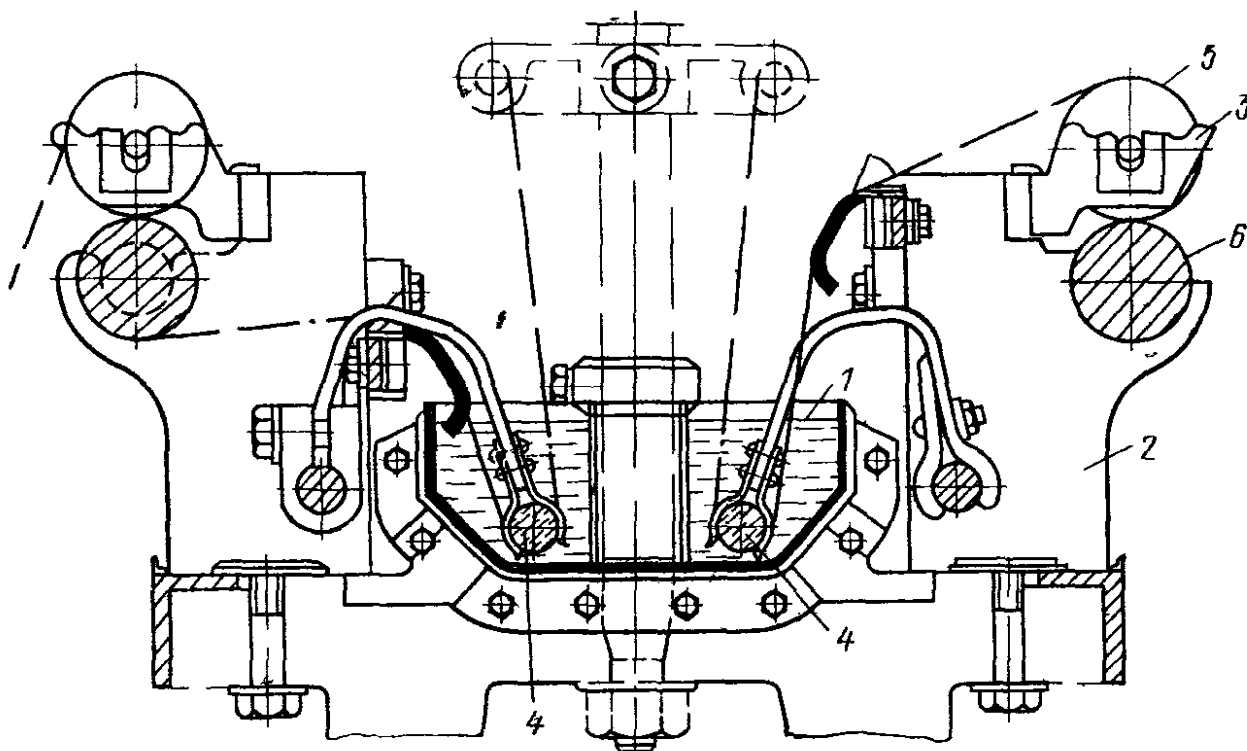
Рисунок 17 - Выпускной прибор кольцевкрутильной машины КМ-83-1ТМ мокрого кручения
